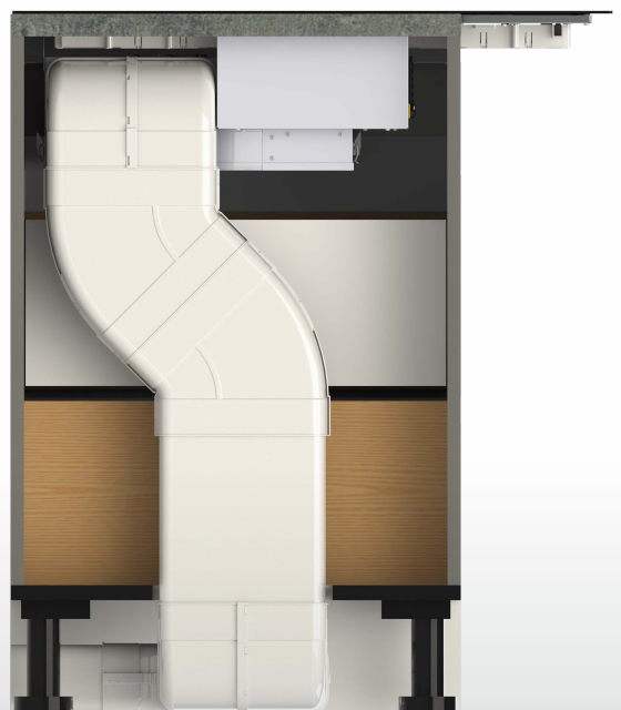
Schacht gebogen, Schrankbreite min. 60 cm
